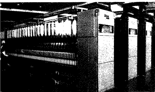
北京第二棉纺织厂引进成套设备建成的细纺车间
