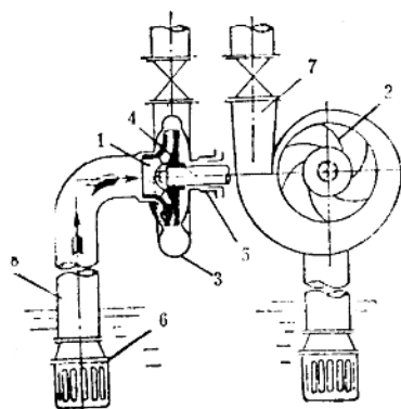
图 1-3 离心泵简图
