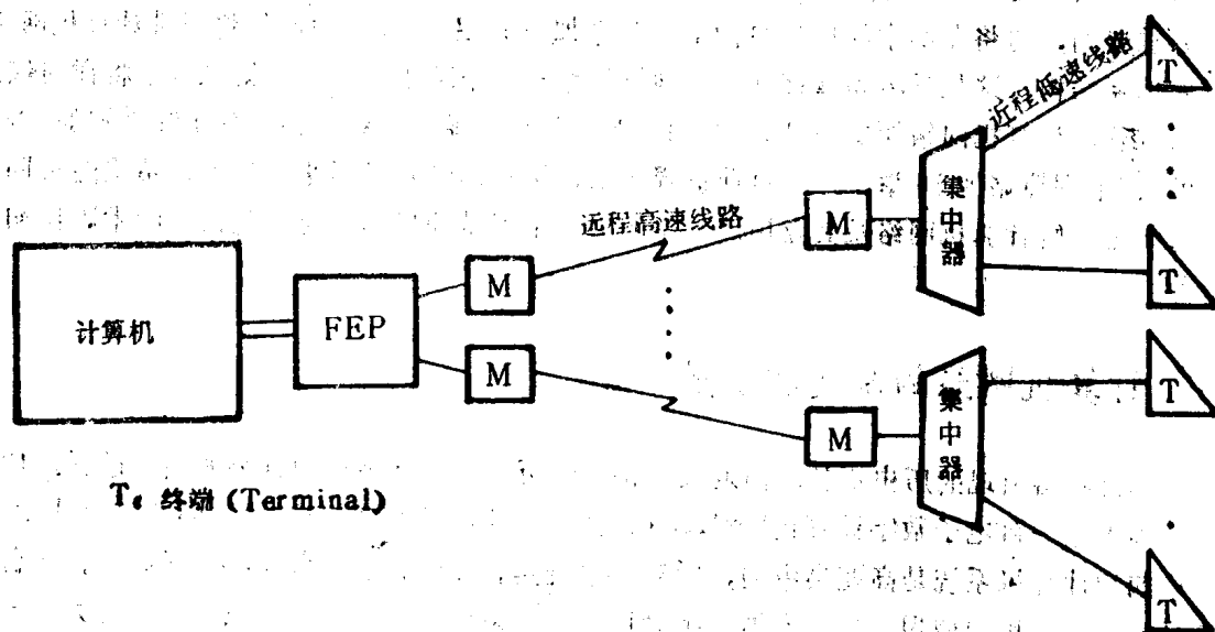
图1.1 以单计算机为中心的远程联机系统
