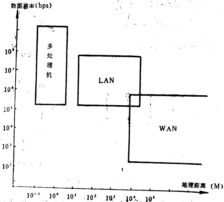
1.4 LAN WAN和多处理机系统的比较
