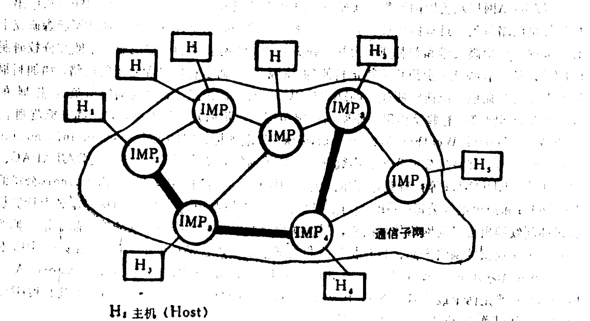
图1.2 存贮转发的计算机网络
