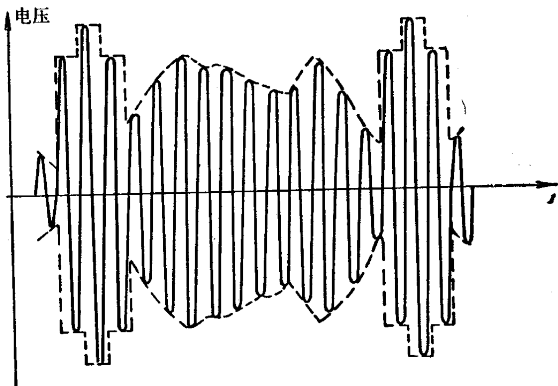
图1-3-1 负极性调制高频信号波形
