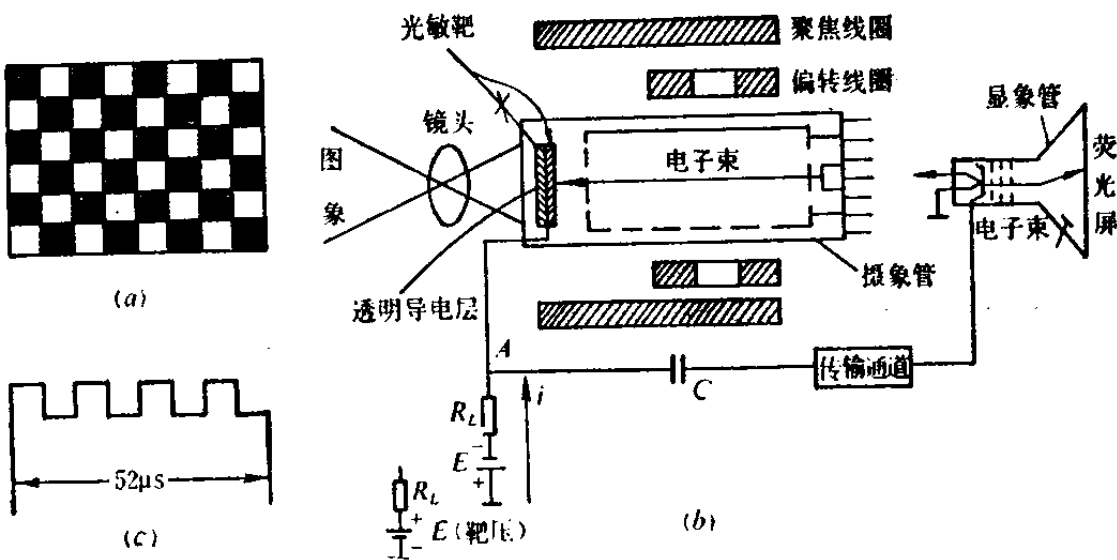
图1-1-1 图象的传送和显示原理
