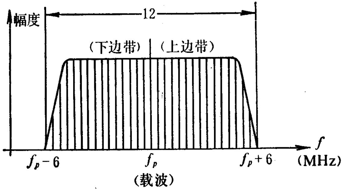
图1-3-2 视频调幅波频谱
