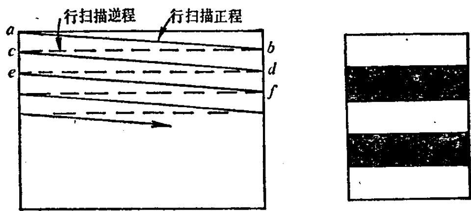
图1-1-2 逐行扫描
