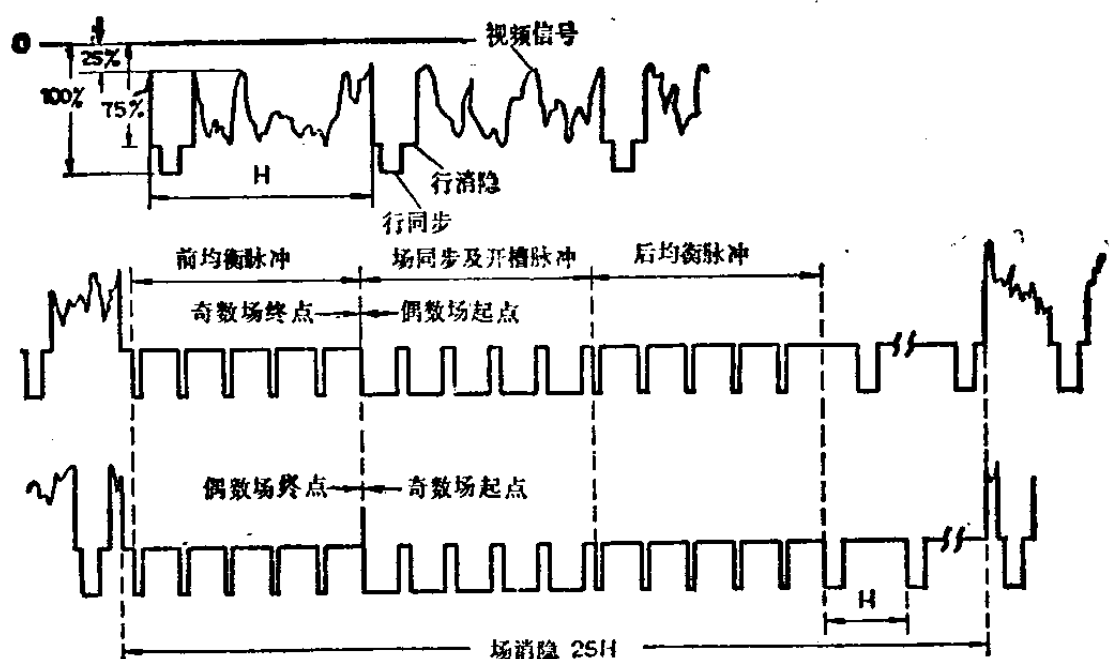
图1-2-1 全电视信号波形图
