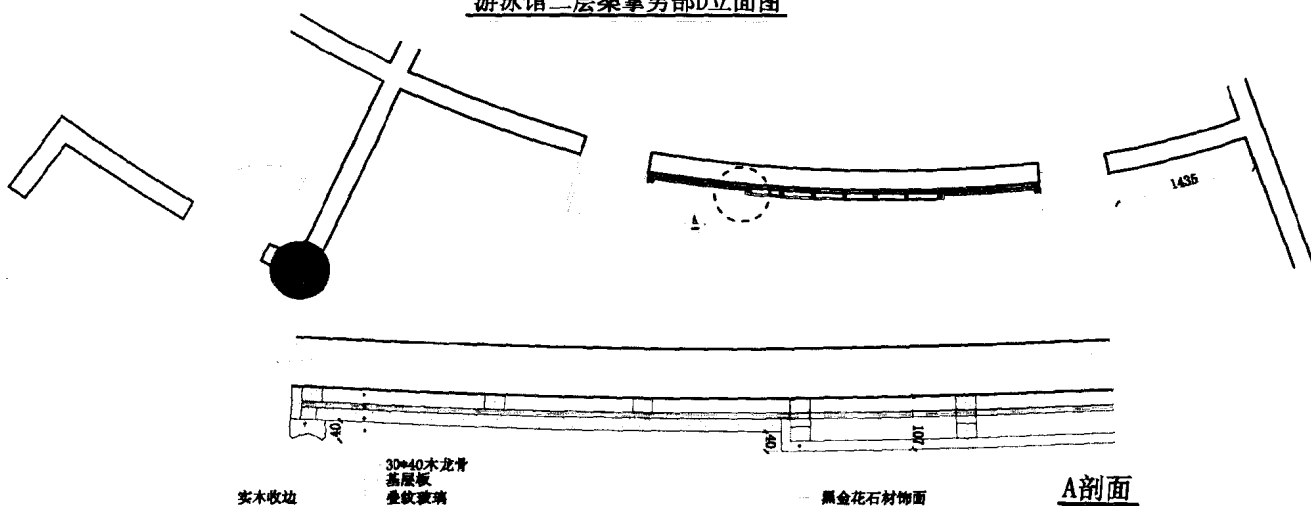
游泳馆二层桑拿男部D立面图
