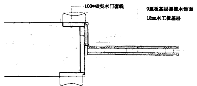
A剖面图
