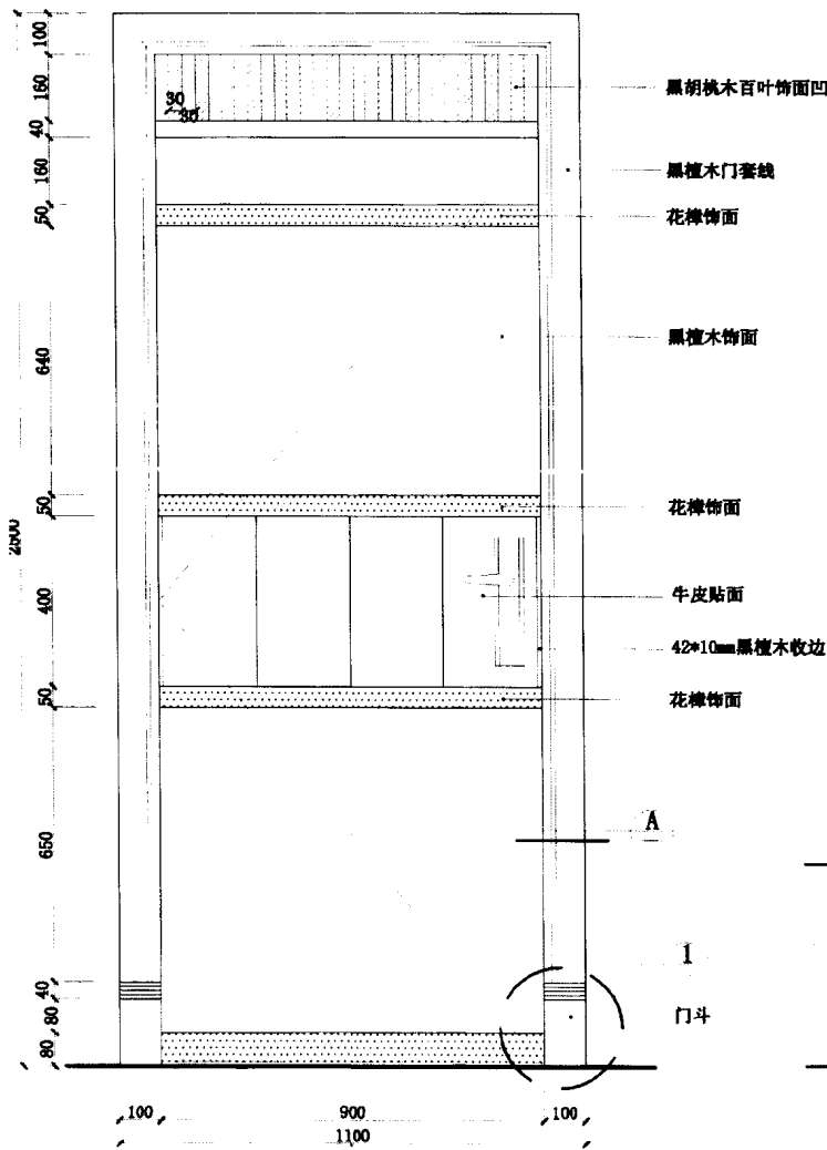
门大样图
