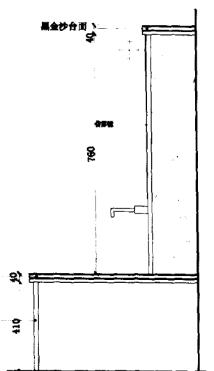
A剖面图
