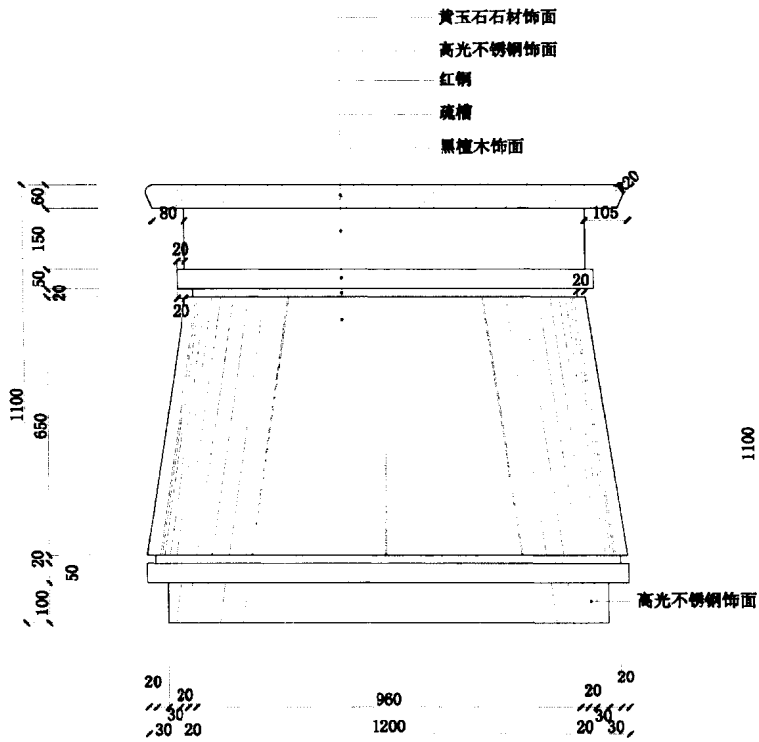
吧台详图
