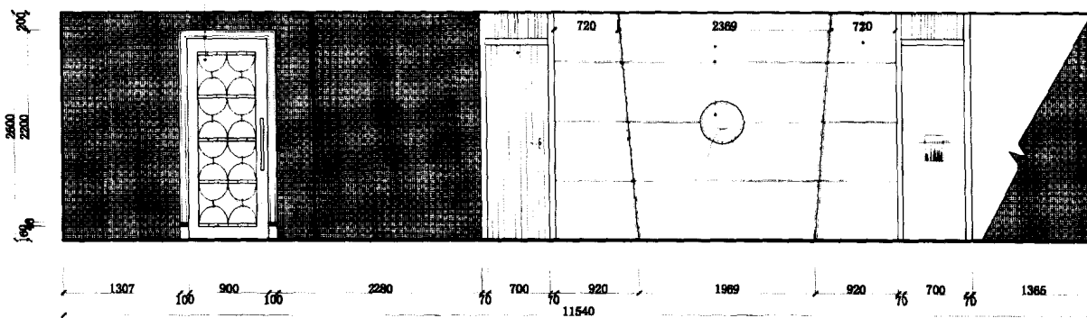
游泳馆二层桑拿男部D立面图
