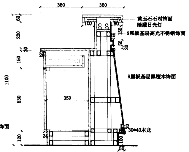
吧台剖面
