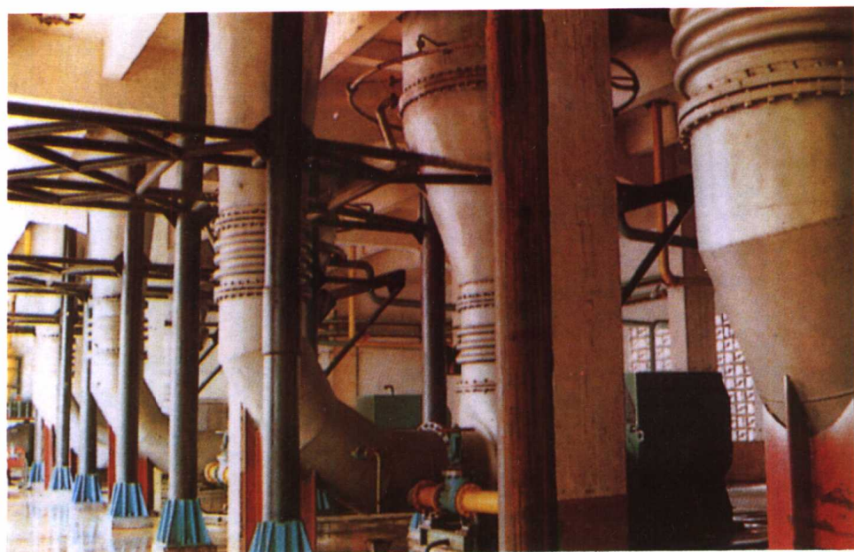
24 湖南省湘澧盐矿年产 20 万吨的真空制盐装置。 (湖南省盐业公司供稿)
