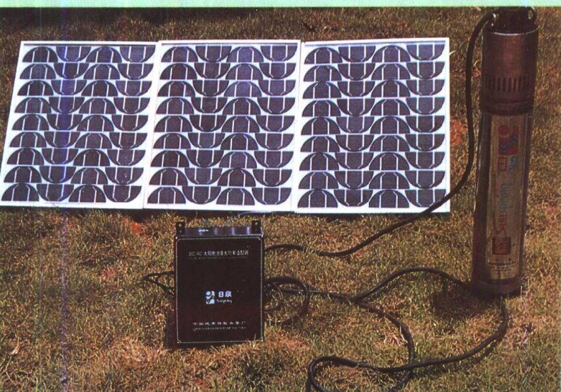
NSP 光伏水泵
