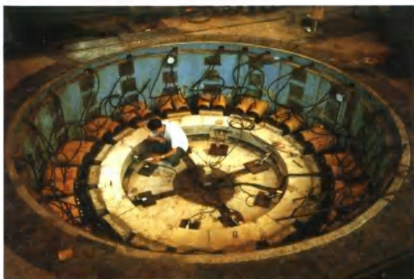
冻结井素混凝土井壁科技成果荣获 1995 年安徽省科技进步二等奖。图为素混凝土井壁模拟试验
