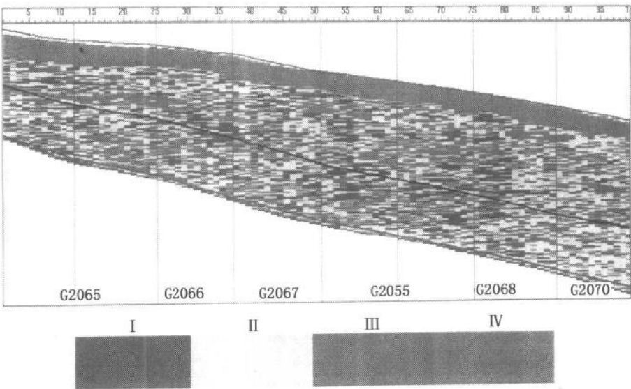
图 8 LINE2 裂缝发育概念模型图
