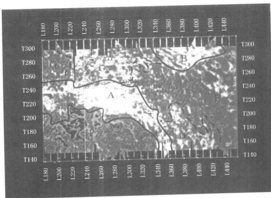
图7 中国西部某油田的均方根振幅属性切片
