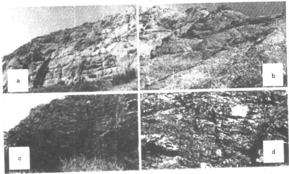
图 1 中国西北部二叠系砂砾岩储层露头裂缝，a 和 b 表示区域性的构造裂缝穿切山体，c 显示垂直缝发育在粗砾岩中，裂缝间距大，d 表示这套砂砾岩储层之下的石炭系板岩中也发育同样的裂缝，均属于区域构造裂缝成因
