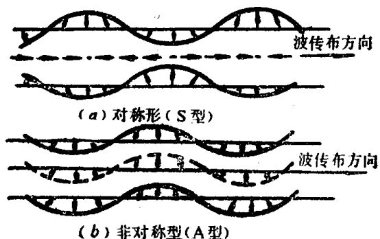
图1.7 兰姆波
