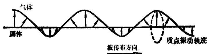
图1.5 表面波（瑞利波）
