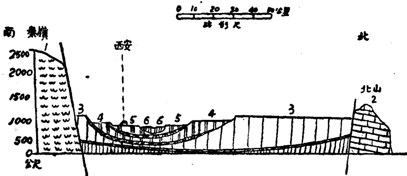
渭河地堑剖面图
