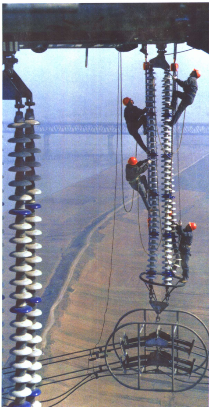
500 千伏洛—平线淮河大跨越施工现场
