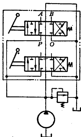
图 7-7 多路阀卸荷回路
