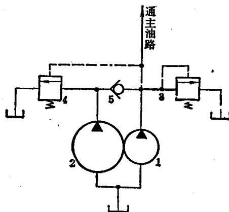
图 7-9 利用卸荷阀的卸荷回路
