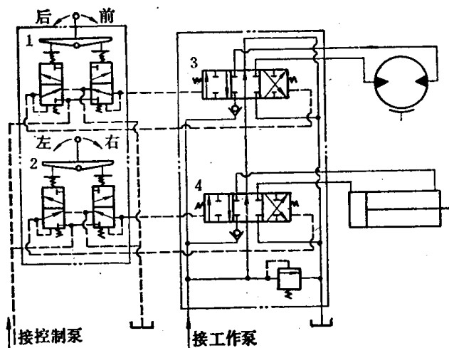
图7-20 使用减压阀式先导换向阀调速回路
