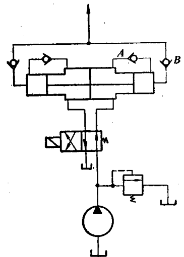
图7-5 连续增压回路
