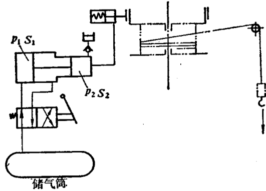
图7-4 间歇增压回路
