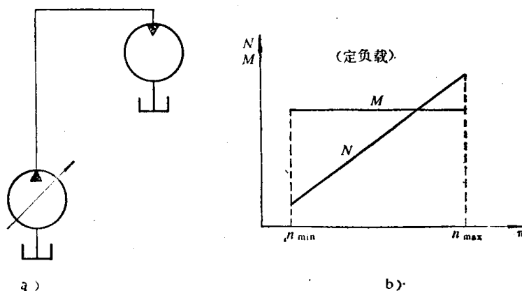
图7-21 变量泵一定量马达调速回路
