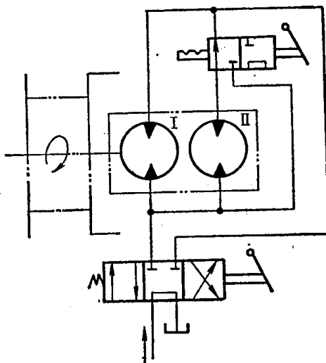
图7-16 有级变量马达调速回路
