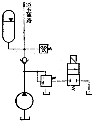
图7-10 利用蓄能器保压的卸荷回路
