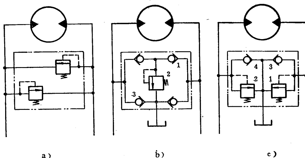
图7-12 采用缓冲补油阀的回路
