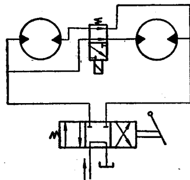
图7-15 定量马达组调速回路
