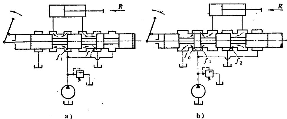
图7-18 使用手动换向阀调速回路
