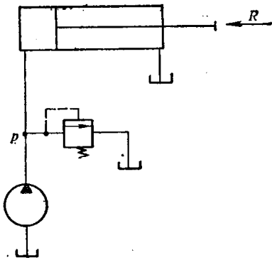
图7-1 单级调压回路
