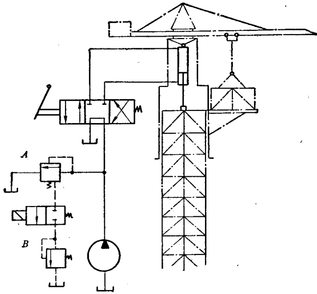
图7-2 两级调压回路
