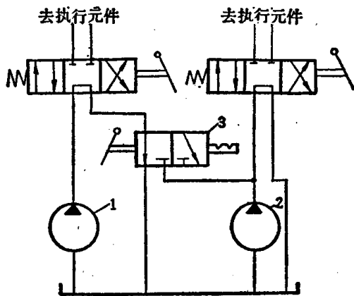
图7-14 定量泵组调速回路
