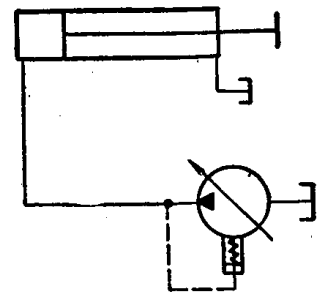
图7-11 利用限压式变量泵保压卸荷回路
