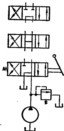
图 7-6 利用滑阀机能卸荷
