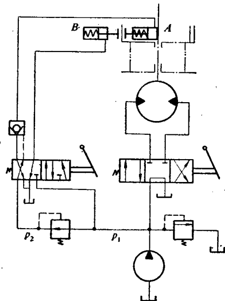
图7-3 用减压阀减压回路
