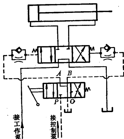
图7-19 使用节流式先导换向阀调速回路
