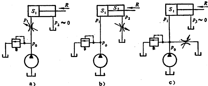
图7-17 节流阀调速回路
