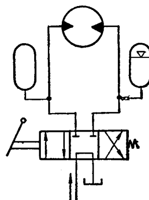
图7-13 采用蓄能器缓冲补油回路
