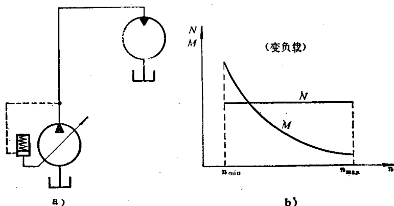
图7-22 恒功率变量泵一定量马达调速回路
