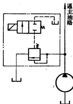
图 7-8 利用电磁溢流阀卸荷回路
