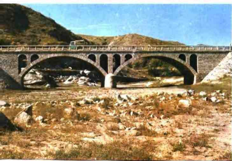
13 西李庄~上连庄公路上重要桥梁——泉河桥，长52米
