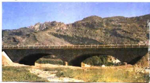
9 阜公路两岭口悬链线石拱桥，3孔，跨径13米， 全长54.955米
