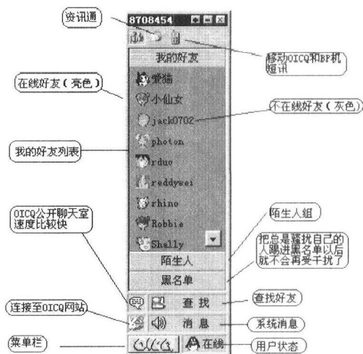
图 1-11 OICQ 使用界面
