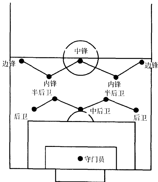
图3 WM阵型
