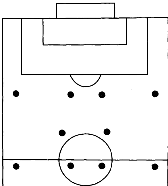
图4 4-2-4阵型
