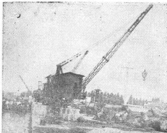
照片5 京杭运河苏北段一期整治工程中兴建的淮阴南港客货运码头
