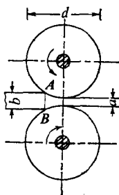
图 3. 轧钢。
