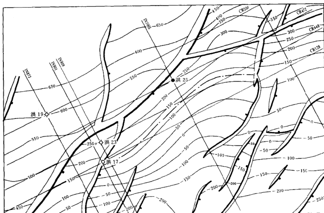
图 1 洪 17 断块 T_6 反射层构造图
