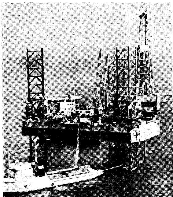
图1-1-1 麦尔斯克勘探者号自升式钻机平台
