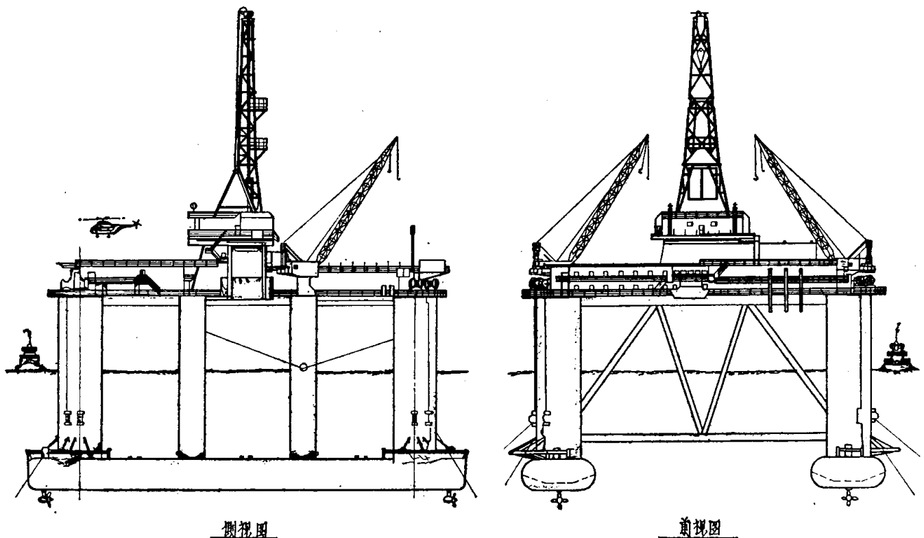
图1-1-4 赛达柯704号半潜式钻井平台
