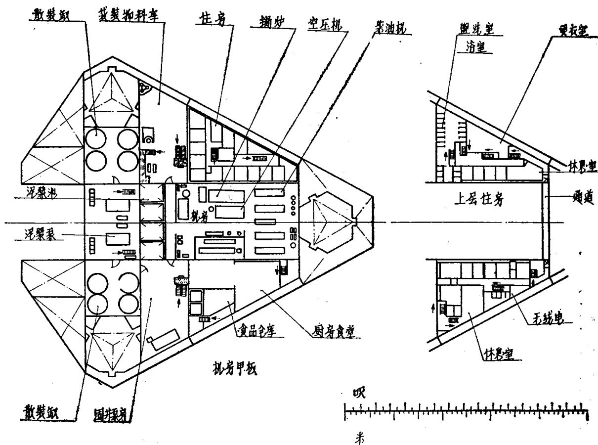
图1-1-3 麦尔斯克勘探者号机房甲板总体布置
