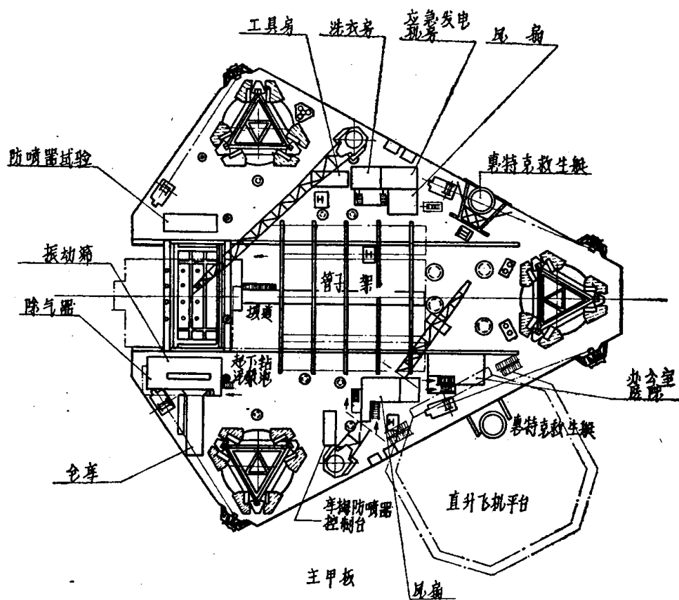
图1-1-2 麦尔斯克勘探者号主甲板总体布置
