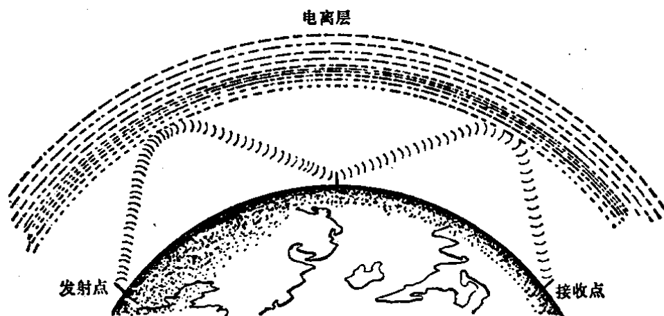
图 1-3 天波
