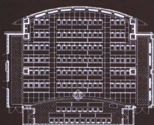
会议厅平面
