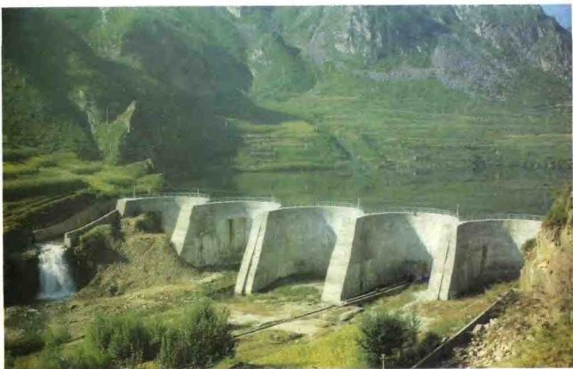
杨树湾连拱坝
