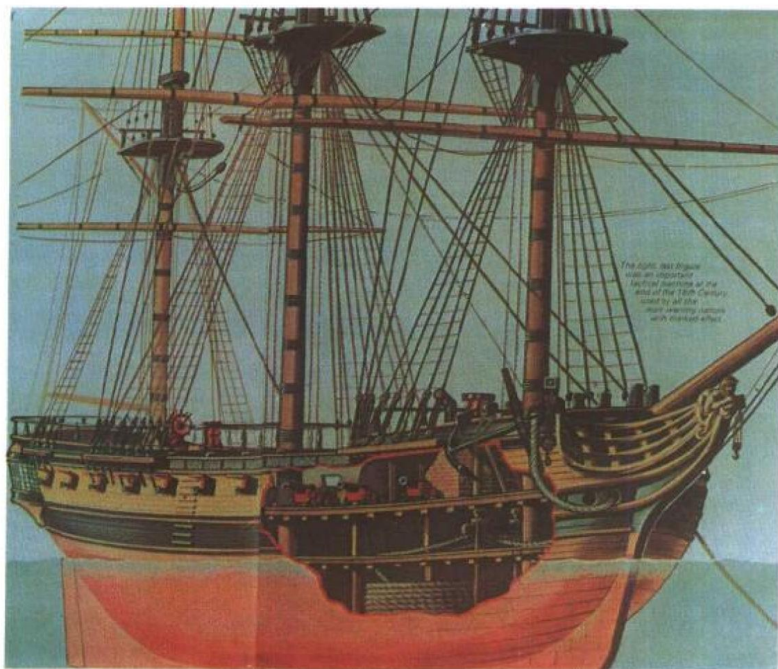
图 17 18 世纪三桅快舰的解剖图。注意从两舷升向桅杆的绳梯。
