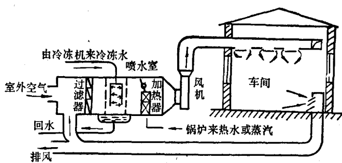
图 0-2 空气调节系统
