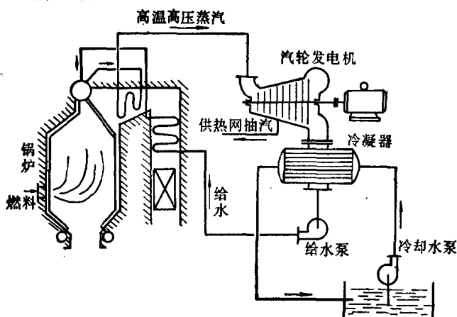
图 0-4 蒸汽动力循环
