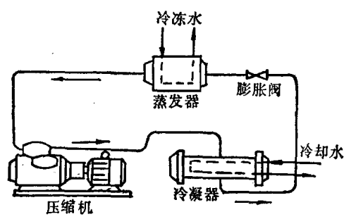
图 0-3 压缩蒸气制冷系统
