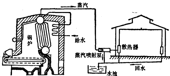
图 0-1 蒸汽喷射热水采暖系统
