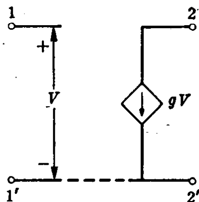
图 7-1 理想电压控制电流源的示意图
