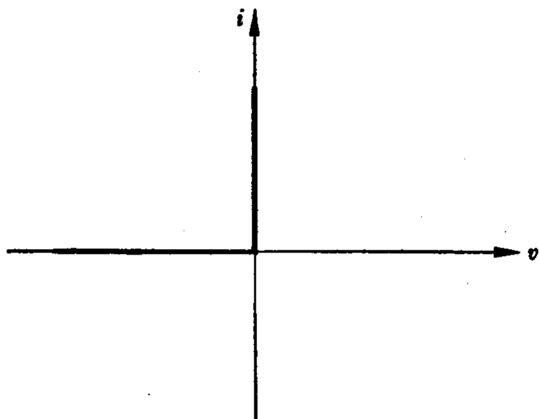
图 7-7 理想二极管的伏安特性
