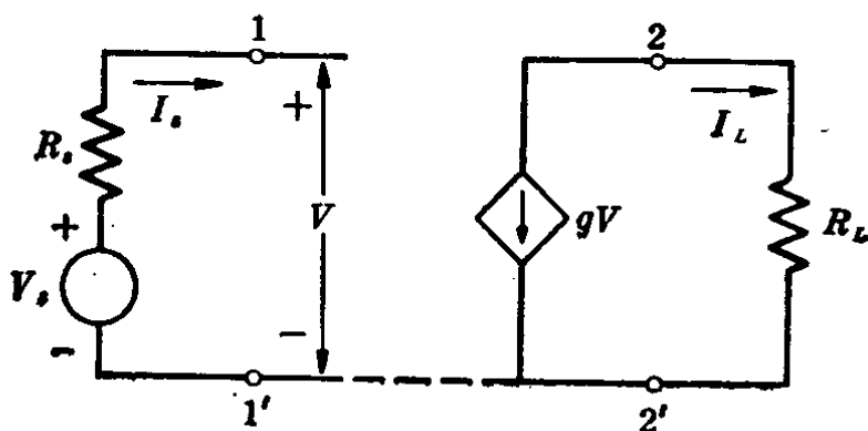
图 7-3 有激励和负载的电压控制电流源
