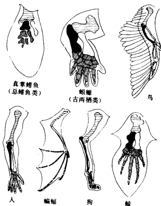
图绪-1 前肢骨的同源
