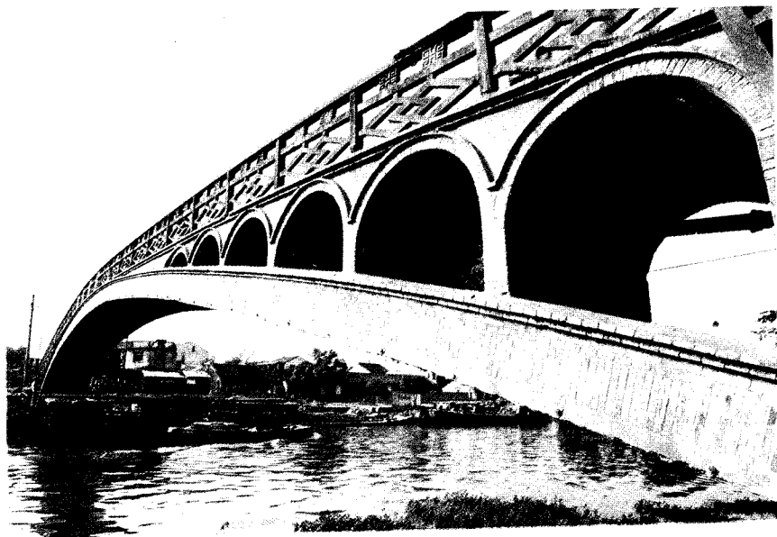
一九六五年建成单孔净跨55米双曲拱胡埭大桥
