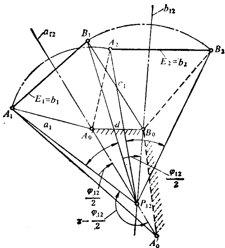
图6.1-5 利用连杆平面实现预期两变位。极与引线间的夹角关系
