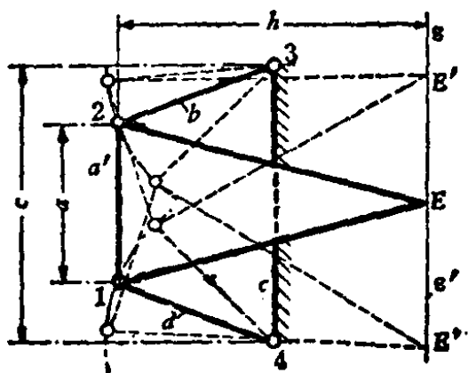
图6.1-2 按照点位设计机构的例子。罗伯次近似直移机构
