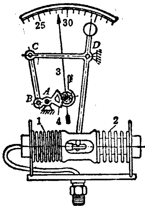
图6.1-4 按照相应角移量设计机构的例子。精密气压表
