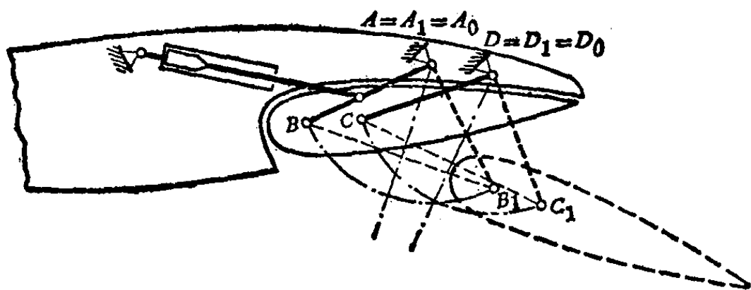
图6.1-3 规定运动杆两位置设计机构。飞机的襟翼机构
