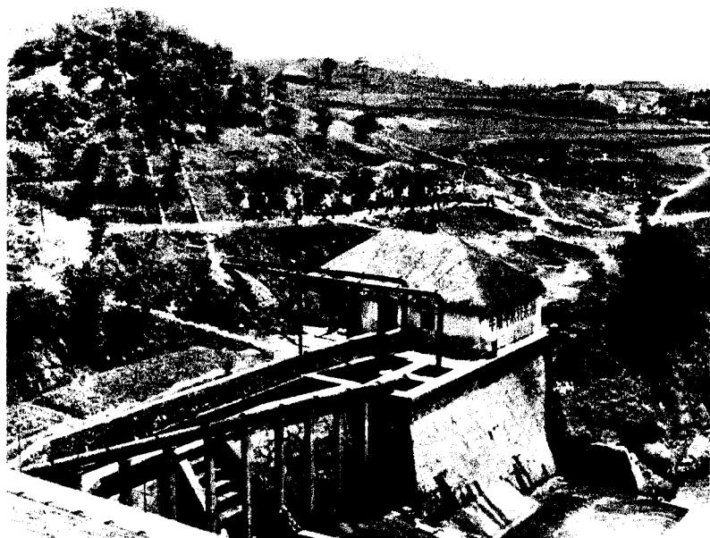
山区人民因地制宜兴办的小型水轮泵站。
