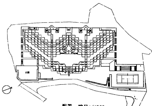
配置 縮尺1/1800
