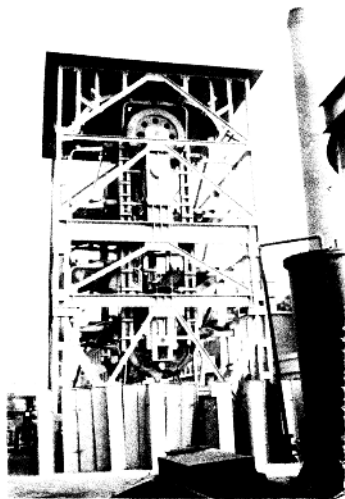
► 承德市经济技术开发总公司所属京承科工联合机械总厂引进消化西德技术生产的垂直式立体车库。
