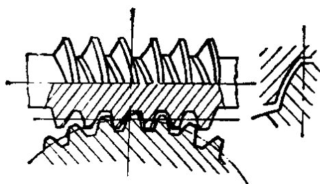
图5-2-5 圆弧齿圆柱蜗杆传动
