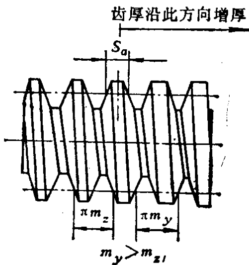
图5-2-6 双导程蜗杆
