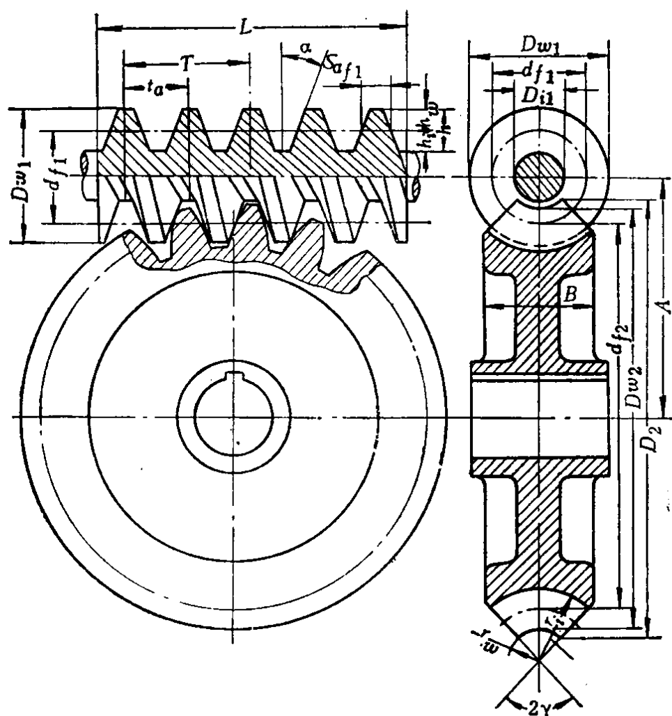
图5-1-1 蜗杆传动啮合图
