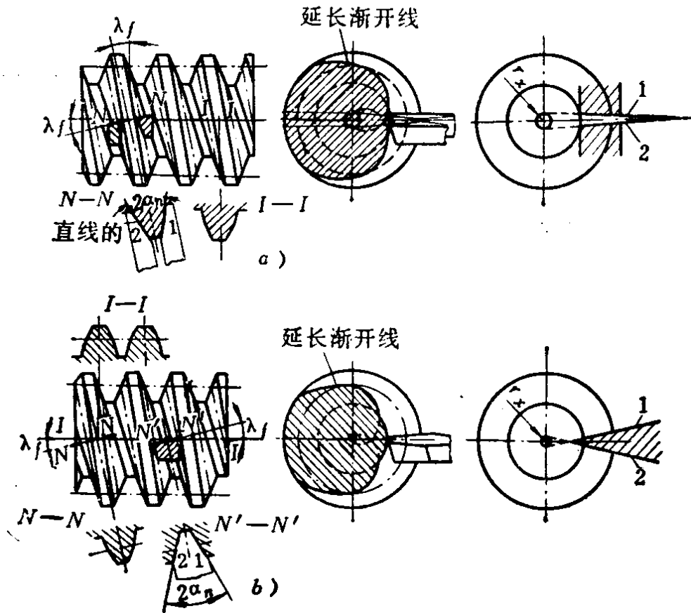
图5-2-2 延长渐开线蜗杆
