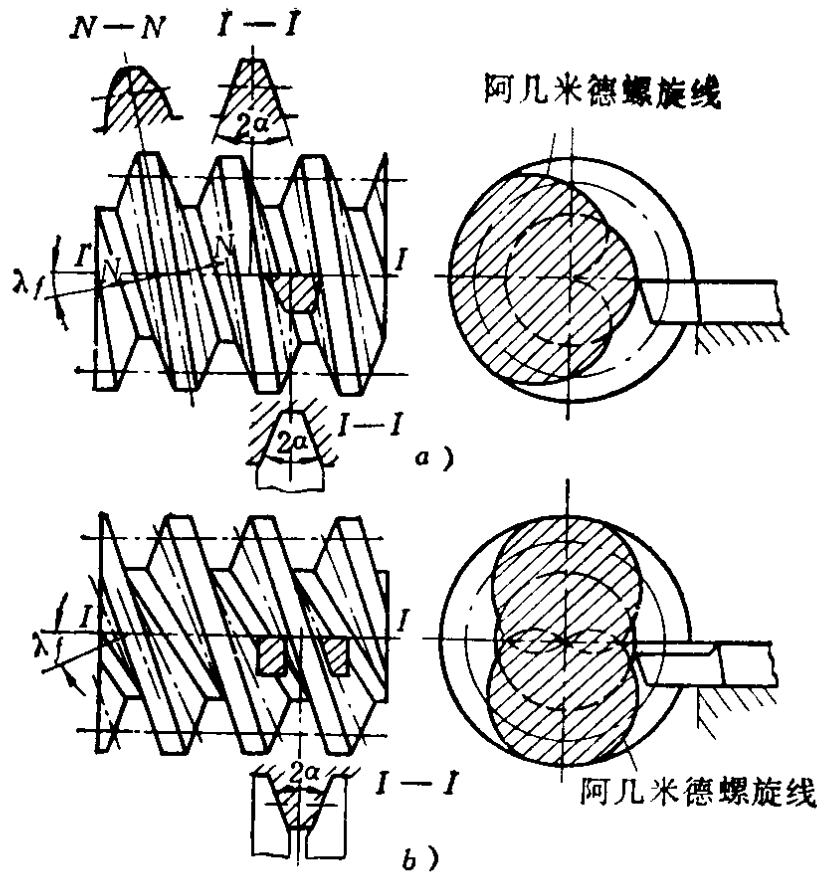
图5-2-1 阿基米德螺旋线蜗杆
