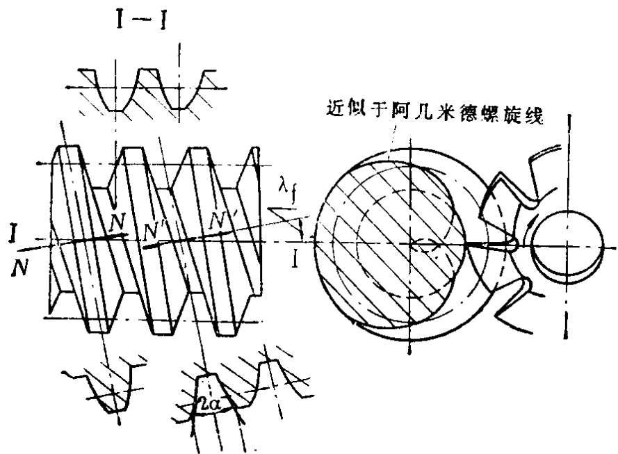
图5-2-4 盘铣刀或砂轮磨削的蜗杆
