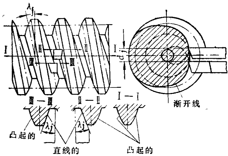
图5-2-3 渐开线蜗杆
