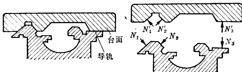
图 1-15 车床台面与导轨
