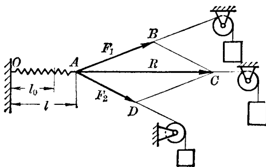
图 1-7 力的平行四边形法则演示
