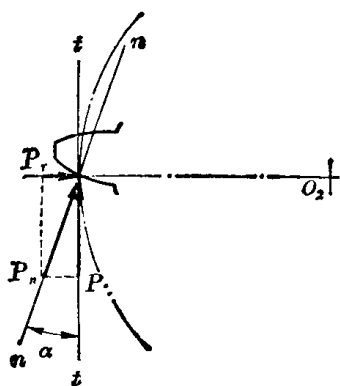
图 1-16 圆柱正齿轮啮合力分解为圆周力和径向力
