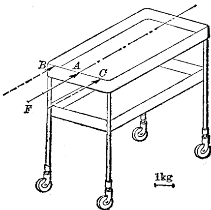
图1-3 力的图示
