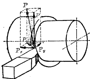
图 1-10 车刀切削工件时切削力的分解
