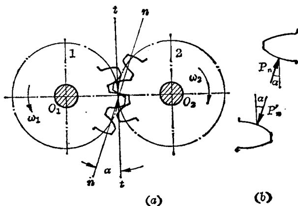
图 1-5 齿轮啮合时的作用力和反作用力
