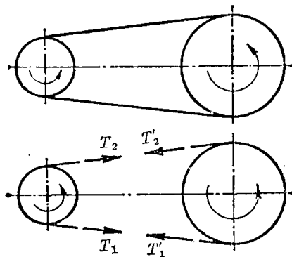
图 1-13 皮带张力
