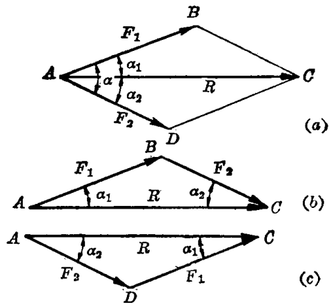
图 1-8 力的平行四边形法则
