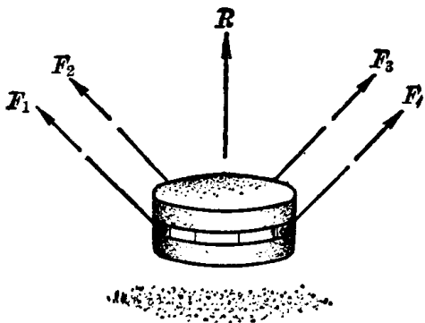
图 1-6 打夯时力的合成
