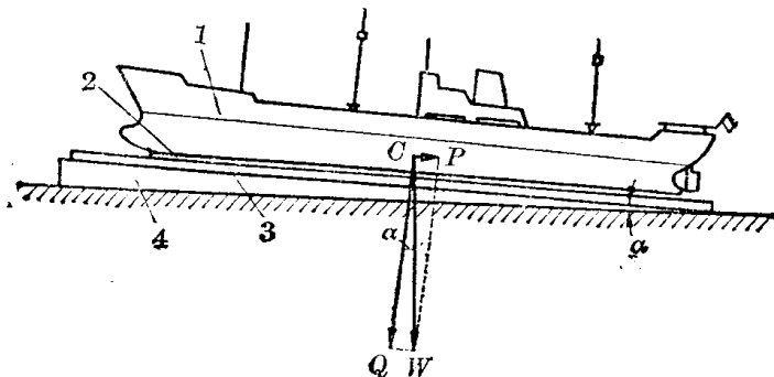
图 1-9 船下水时重力的分解
