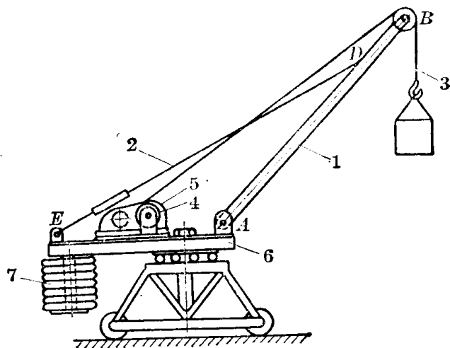
图 1-11 起重机
