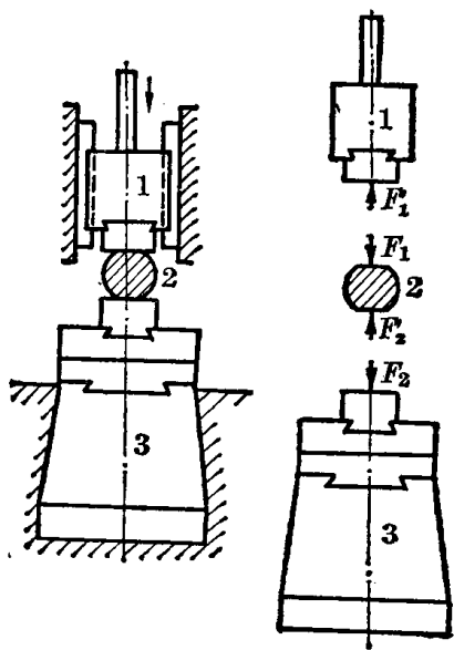
图 1-4 锻压时工件的作用力和反作用力
