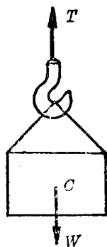
图 1-12 钢丝绳拉力
