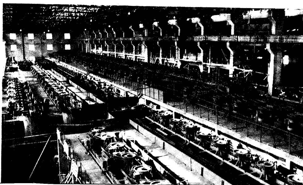
落雪矿选厂浮选车间
