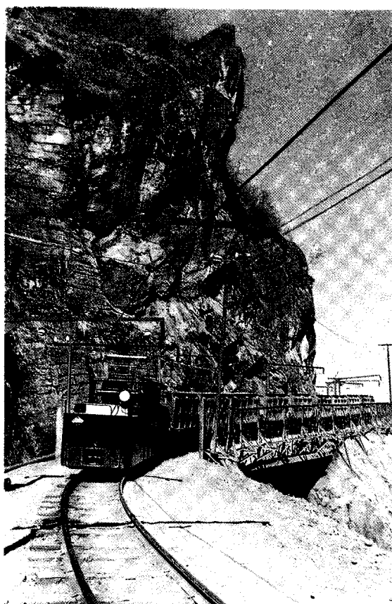
铜矿石运输线
