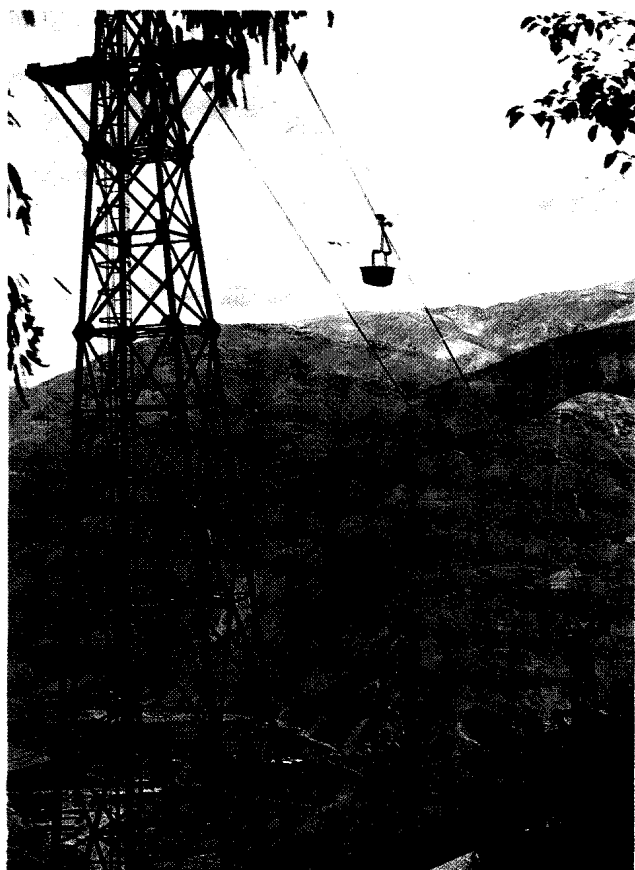
汤丹矿运矿索道
