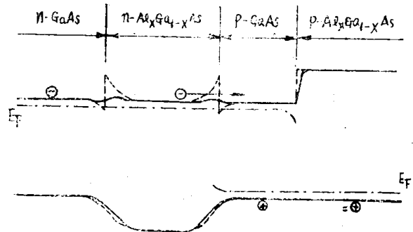
图 9 \text{GaAs}-\text{Al}_x\text{Ga}_{1-x}\text{As} 的 n-n, n-p, p-p 异质结的能带图。p-n 结加正向偏压。——实变法, ————缓变法, - - - - 费米能级。
