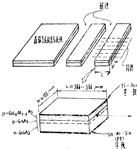
图17 激光二极管的切割与解理过程
