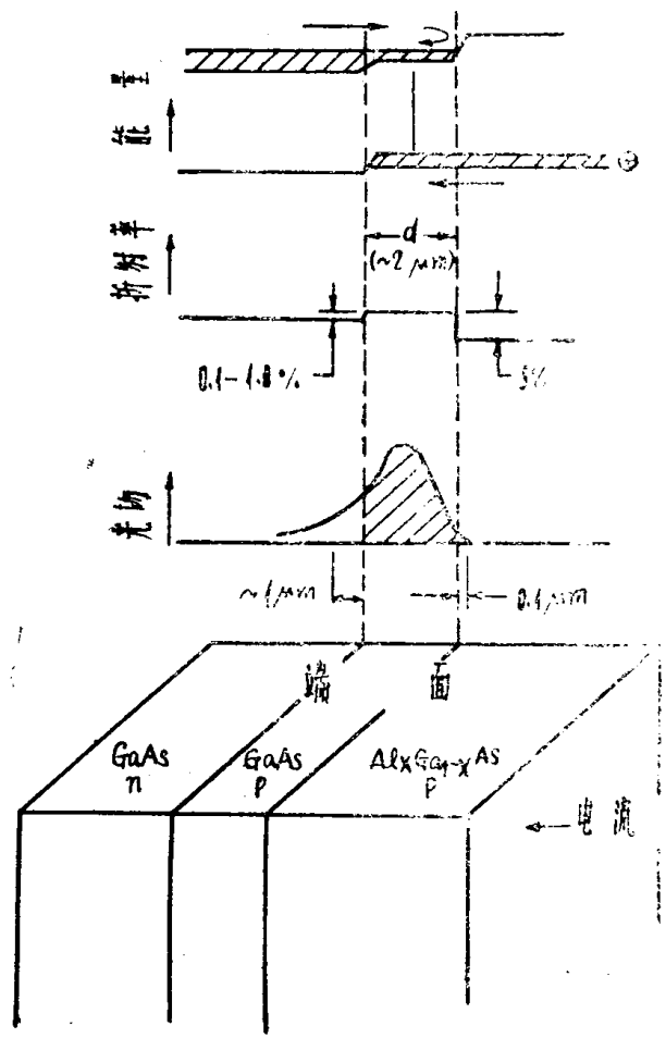
图 14 单异质结构激光器的能带图，折射率，光场分布和物理结构。
