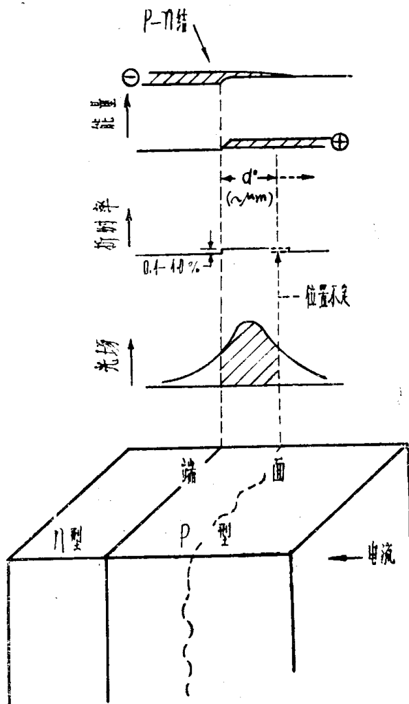
图2 加正向偏压的扩散同质结构激光二极管的带边, 折射率和光场分布的示意图。为了说明问题, 有源区右边位置的不确定性和不规则程度已被夸大。加大正向偏压的能带图如上方所示, n区和p区都是简并掺杂的。电子注入到p区, 而空穴的注入可以忽略不计。注入电子的数目很大, 足以使 d_0 区中电子和空穴的准费米能级差满足条件 F_c - F_v > h\nu 。
