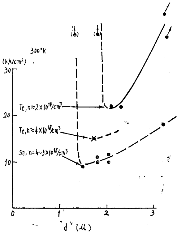
图20 在300K下，用掺杂不同的衬底制作的几个法布里—珀罗型SH二极管(腔长400—500 \mu )的 J_{th} 与 d 的关系。引自文献(23)。
