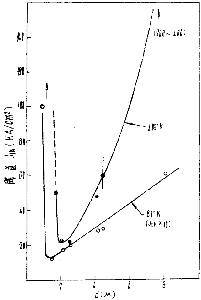
图19 在 300\text{K} 和 80\text{K} 下, 无涂层的法布里-珀罗型 SH 二极管的 J_{th} 与 d 的关系。这里所有的二极管都是在掺 \text{Te } 2 \times 10^{18} / \text{cm}^3 的 GaAs 上制作的。引自文献(23)。
