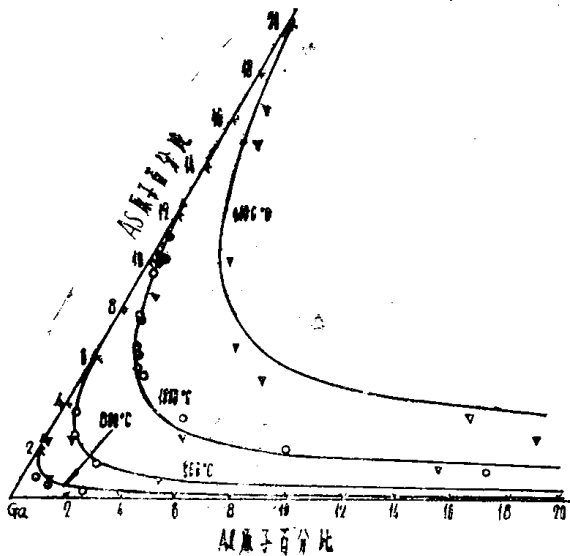
图4 Al-Ga-As相图中Ga角液相等温线的细节。△文献[20], ○文献[25], ●文献[26]。
