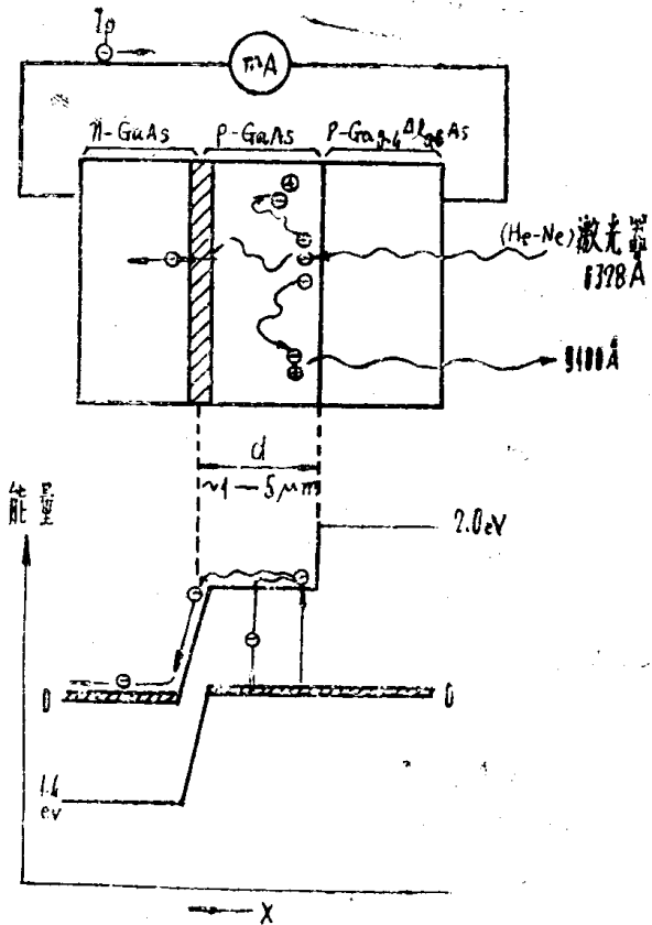
图11 证明 GaAs—Al x Ga 1-x As 异质结界面没有陷阱测量方法的示意图。引自文献[23]。
