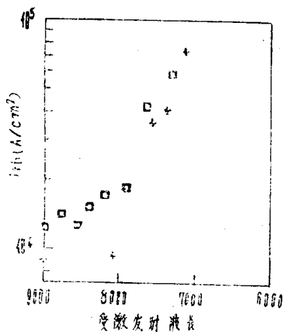
图16 在300K下，有源区为Al x Ga 1-x As的SH激光器的受激发射阈值电流密度与受激发射波长的关系。□文献[40]，×文献[41]。
