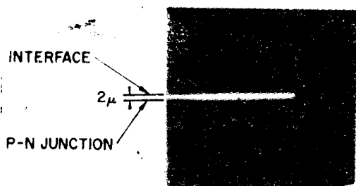
图18 SH二极管端面的自发发射光:(a)10KA/cm², (b)27KA/cm²。引自文献[23]。
