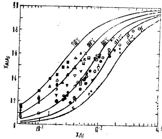
图6 Al-Ga-As系的固相等温线。由一个元素的组分 X_{Al} 规定溶液的组分, 因为在图5中已经给出了液相等温线。实际上可以认为液相线指的是Al在用As或GaAs饱和的Al-Ga溶液中的原子百分比。□, ×, ●和I分别为700°, 800°, 900°和1000°C [28] ; ▣, ▢和⊖分别为800°, 850°和900°C [25] ; ○为1000°C [25] ; ▫为1000°C [20] ; ■为707°C, △为756°C, ▲为802°C, ▽为852°C, □为900°C, ●为970°C, ▼为1020°C, +为1060°C [26] 。实线是根据实验数据通过简单的计算估计出来的。
