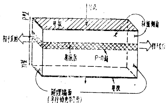
图1 具有法布里-珀罗腔的同质结构激光器。
