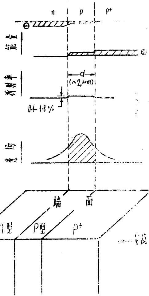
图3 加正向偏压的液相外延同质结构激光器的带边，折射率和光场分布的示意图。引自文献[12]。
