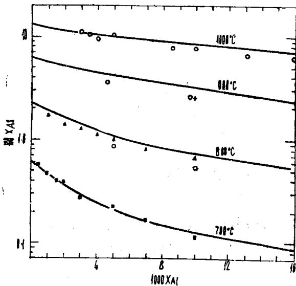
图5 Al-Ga-As系的液相等温线。+ 900°和1000°C [20] , ○800°, 900°和1000°C [25] ■712°C, ▲802°C, ▼1000°C, 实线是根据实验数据通过简单的计算估计出来的。
