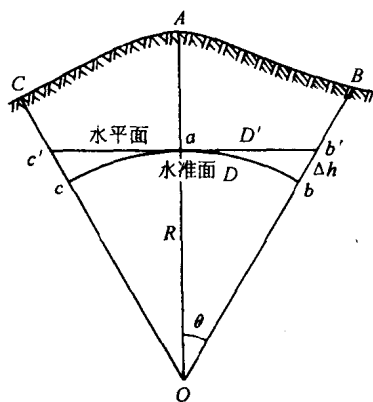
图 1-5 地球曲率对水平距离和高程的影响
