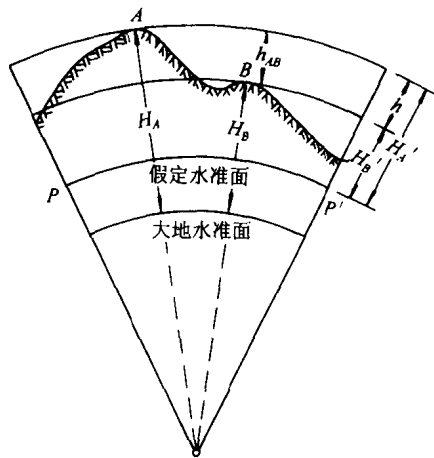
图 1-10 高程表示
