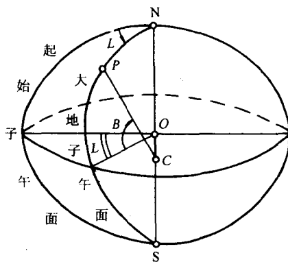
图 1-7 大地坐标系
