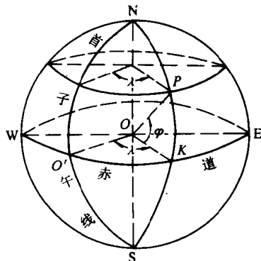
图 1-8 天文坐标系
