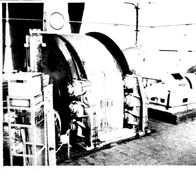
主井绞车房
