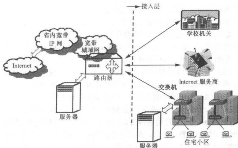
图 1-1 一种宽带接入解决方案
