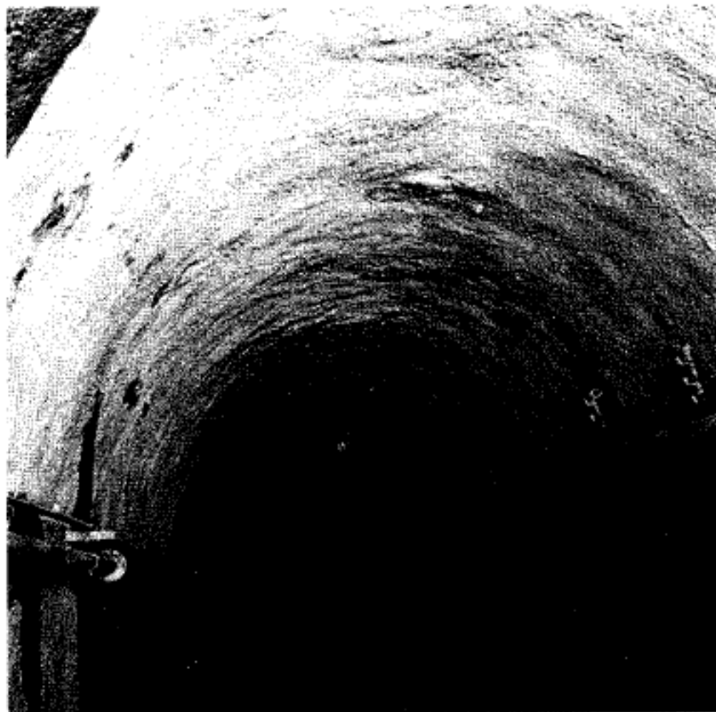
岩巷光面爆破锚杆砼喷浆联合支护巷道
