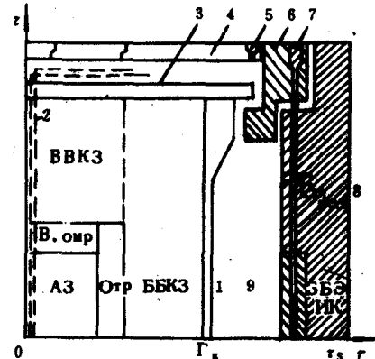
图 15.1 动力反应堆屏蔽上半部有效区段的布置简图
