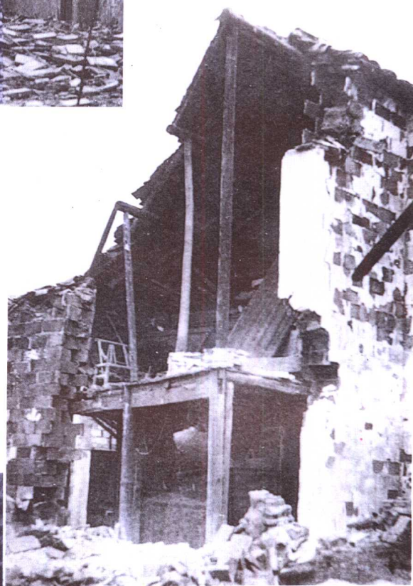
溧阳上沛民居两层楼房墙体垮落，木柱 歪斜。
