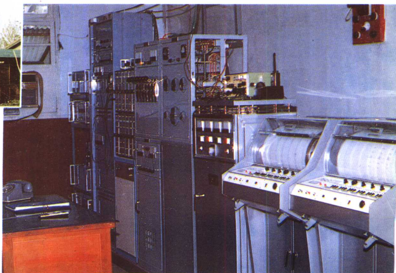
南京遥测地震台网南京记录中心机房。
