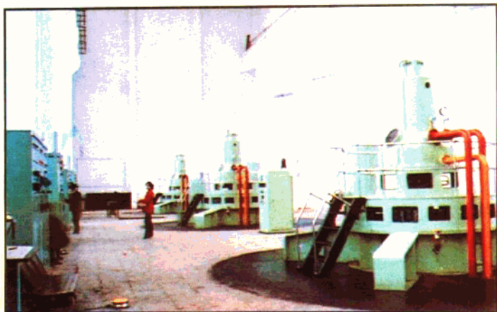
支持能源工业发展——潭家堰电站发电机组
