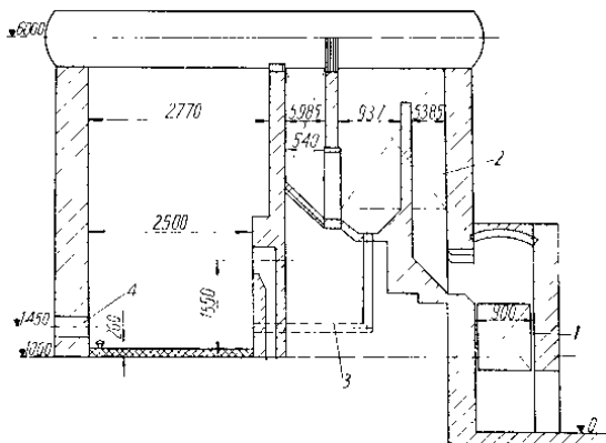
图 1-3 武汉制氮厂沸腾炉示意图
