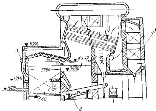
图 1-2 广州糖厂沸腾炉简图
