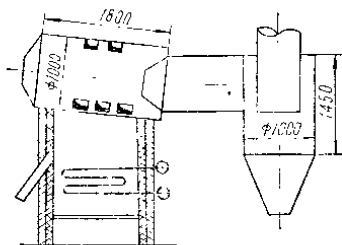
图 1-4 带卧式旋风燃烬室的 4 吨/时沸腾炉试验台
