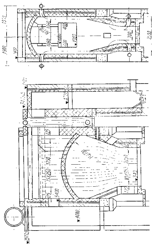
图 1-1 江门肥皂厂蒸汽炉总图
