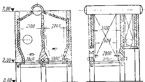
图 1-5 20吨/时双室沸腾炉示意图
