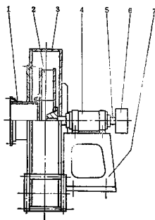
图7-1-2 高压离心通风机
