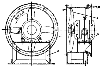
图7-1-3 低压轴流通风机
