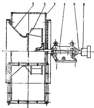
图7-1-1 中低压离心通风机
