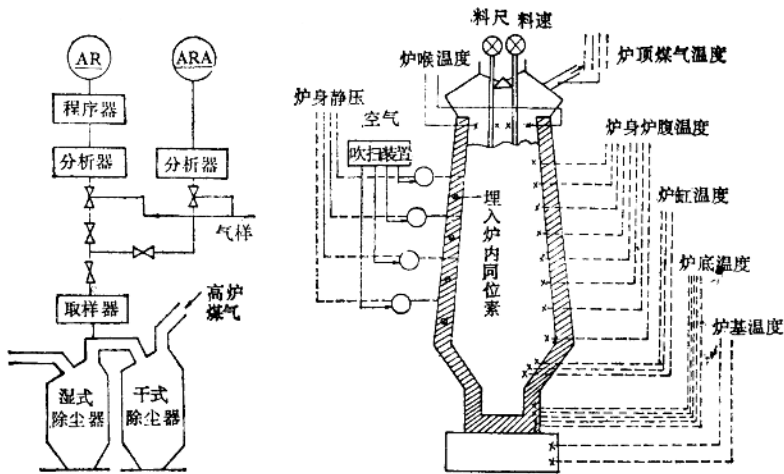
图 1-2 高炉检测参数示意图
