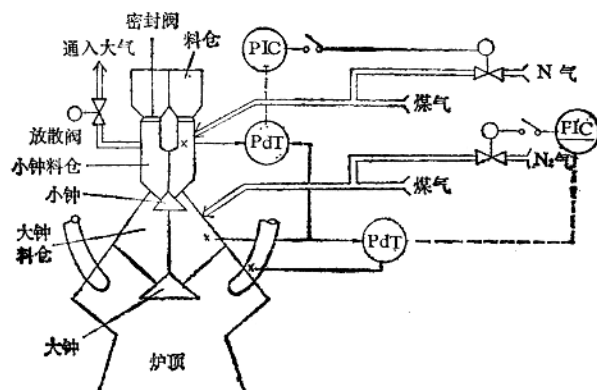
图 1-7 炉顶装料均压控制系统
