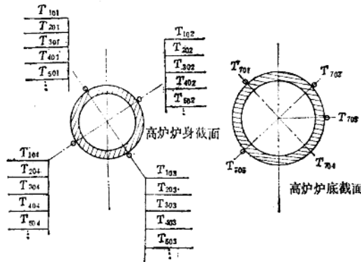
图 1-3 炉体温度检测示意图
