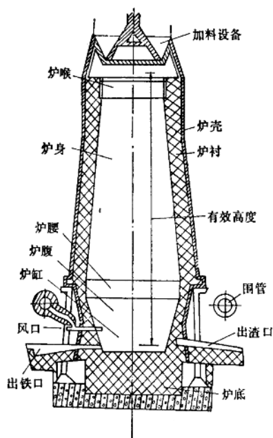
图 1-1 高炉结构简图
