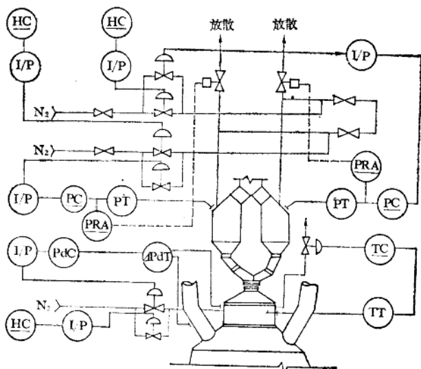
图 1-8 无料钟炉顶均压控制系统
