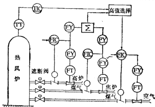
图 1-14 热风炉燃烧控制系统
