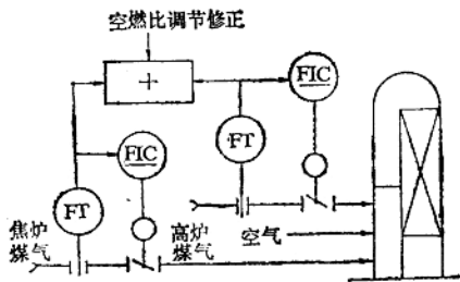
图 1-12 煤气流量控制系统
