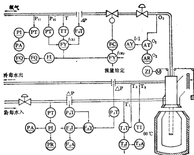
图 1-16 供氧系统自动控制原理图
