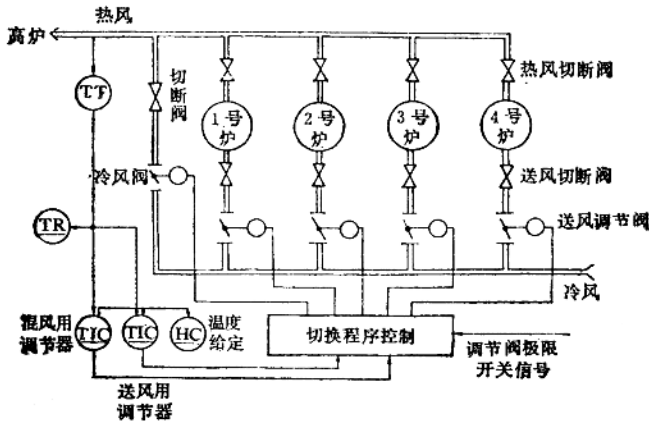
图 1-10 热风温度控制系统
