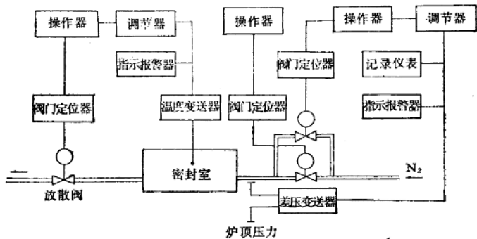
图 1-9 料斗均压控制系统
