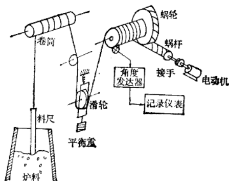
图 1-5 装料深度（料位）测量原理示意图
