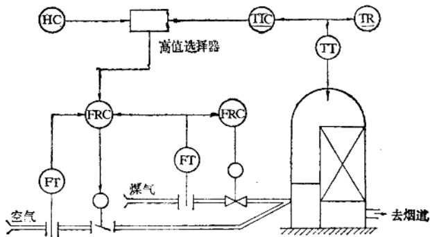
图 1-11 热风炉炉顶温度控制系统
