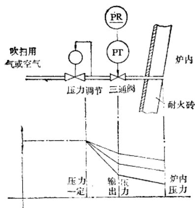
图 1-4 炉身静压测量装置结构图
