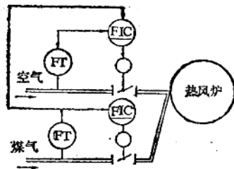
图 1-13 热风炉燃烧用助燃空气流量控制系统
