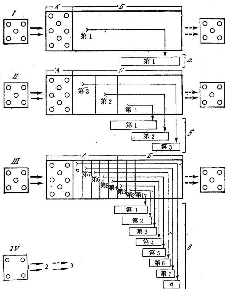
图2 一次(I)、分批(II)和连续(III)产卵类型鱼类诸卵母细胞发育的不同特征。 1——原生质期诸卵母细胞(下一年的一个世代); 2——卵黄发生期诸卵母细胞的生长; 3——产卵后一些吸收过程; A——诸卵母细胞原生质生长期; B——诸卵母细胞营养质生长期; a——短时间产卵期——同步发育的卵母细胞的一次排卵; b——卵黄发生期诸卵母细胞非同步发育和断续排卵的长时间产卵期; B——诸性细胞连续产出的十分长久的产卵期; 某些批卵发育和产出的第1, 2, 3, ..., n特征。
