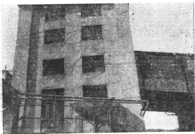
I-2 岩移引起韩城电厂厂房开裂
