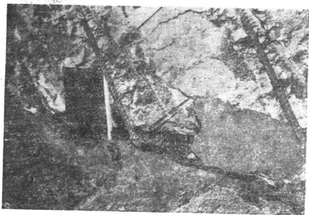
Ⅲ-2 象山煤矿岩移使巷道壁破裂
