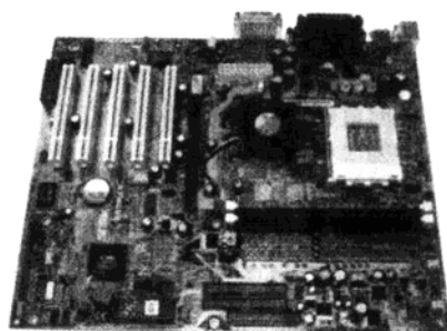
图 1-4 华硕 A7M266 主板
