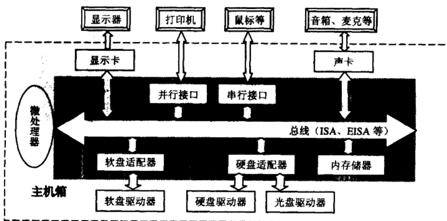
图 1-2 IBM 系列微型机的基本结构
