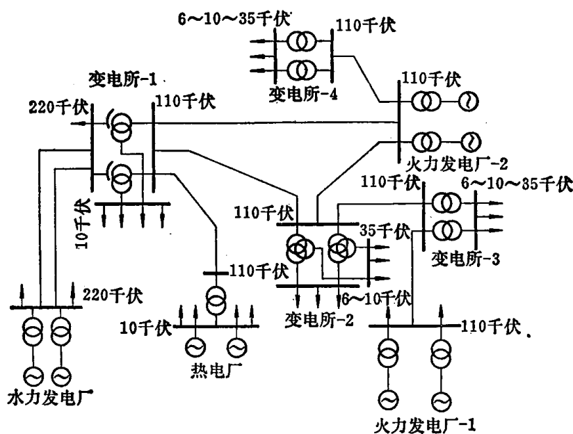
图 1-1 高压电力系统
