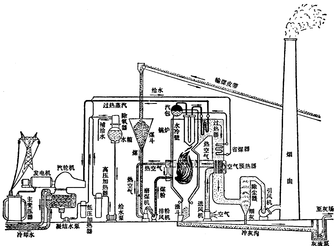
图 1-2 凝汽式火力发电厂生产过程示意
