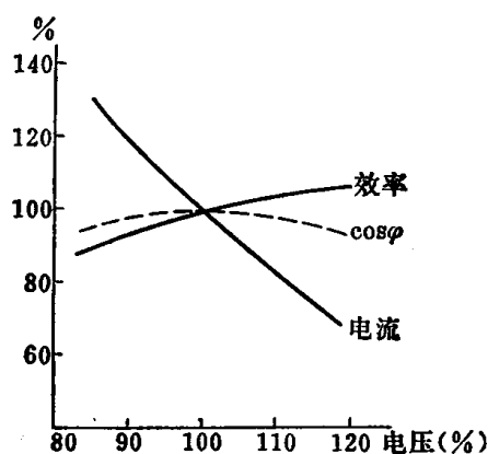
图 1-6 输出功率一定时异步电动机的定子电流、功率因数和效率与电压的关系 (图中的100%表示额定值)
