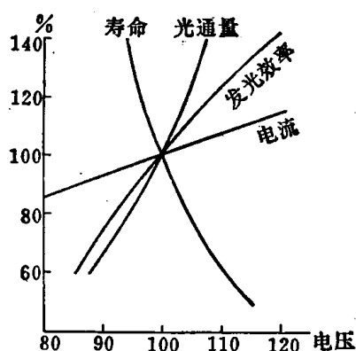
图 1-5 照明负荷（白炽灯）的电压特性
